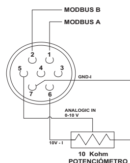
CONECTOR DE ENTRADA/SALIDA
