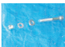
TORNILLO M8x60 TCEI ZN ROSETA 8.4x16 H1.6 ZN TUERCA AUTOBL. M8 ZN
