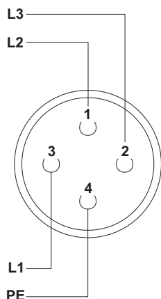
CONECTOR DE ALIMENTACIÓN (TRIFÁSICO)
